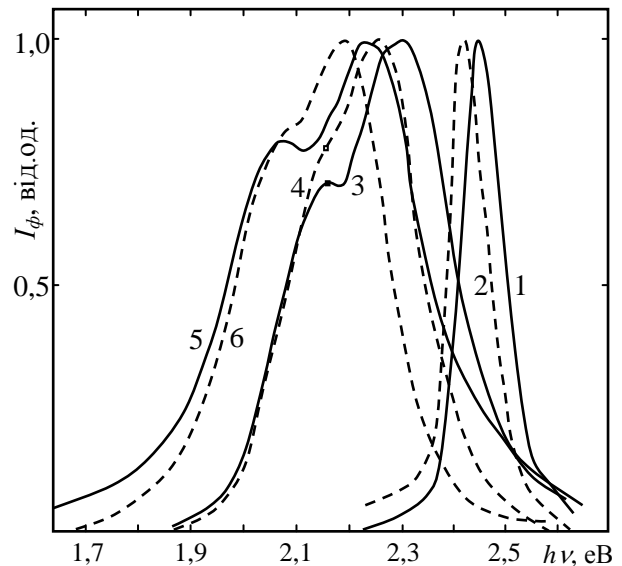
Рис. 1. Поляризовані спектри фотопровідності (1, 3, 5 – E \parallel a , 2, 4, 6 – E \parallel c ) кристалічного \text{SnGeS}_3 , вирощеного при v = 0.1 \text{ мм/год} , виміряні при T , К: 1, 2 – 100; 3, 4 – 293; 5, 6 – 370.
