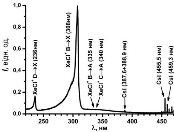
Рис. 3. Інтегрований в часі емісійний спектр ексилампи на суміші Хе-СsСl. Напруга випрямляча 5 кВ, частота 6 кГц, тиск ксенону 30 Тор, температура ГРТ 950 К.
