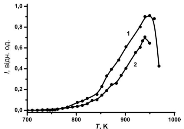
Рис. 4. Залежності інтенсивності випромінювання суміші Хе-СsСl від температури ГРТ на довжині хвилі \lambda=308 нм. Напруга випрямляча 2 кВ, частота 4 кГц, тиск ксенону 45 Тор (1), 75 Тор (2).
