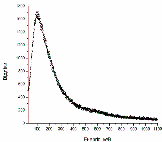
Рис.4. Спектр фону
