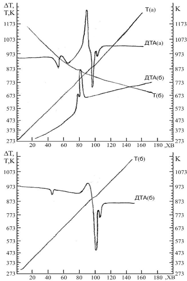
Рис.2 Термограми сплаву \text{Ge}_{0,4}\text{S}_{0,6}\text{-Pb}
