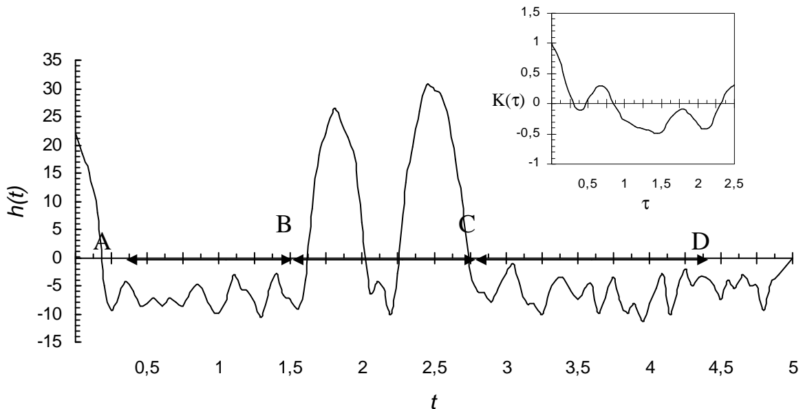
Рис.4. Профіль рельєфу і кореляційна функція для плівок складу Ge_2S_3:Te .
