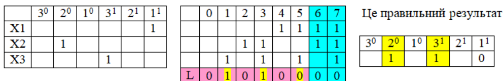
Рис. 14. Моделювання несправностей набору (0 1 0) для шаблону downto
