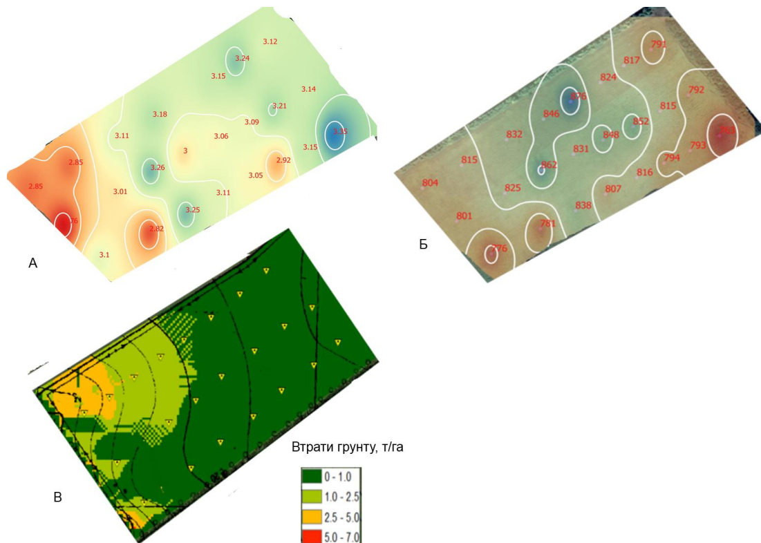
Рис. 2 – Картограми: А – умісту органічного вуглецю, %; Б – питомої магнітної сприйнятливості ґрунту, 10^{-9} м 3 /кг; В – потенційного змиву, т/га
