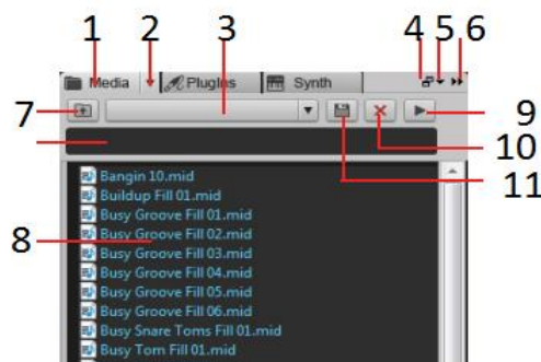
Рис.7.1. Панель Browser
