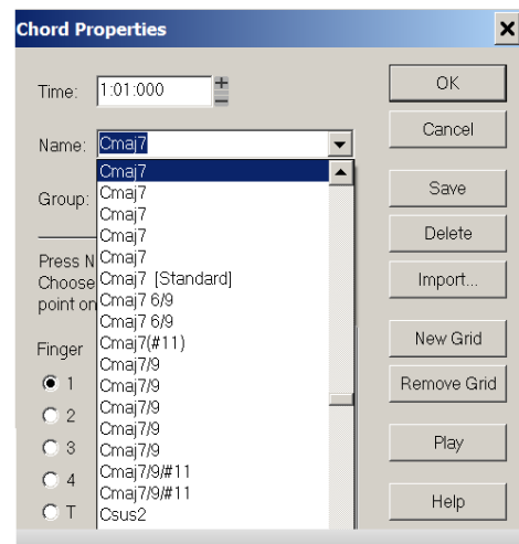
Рис.4.21. Список акордів
