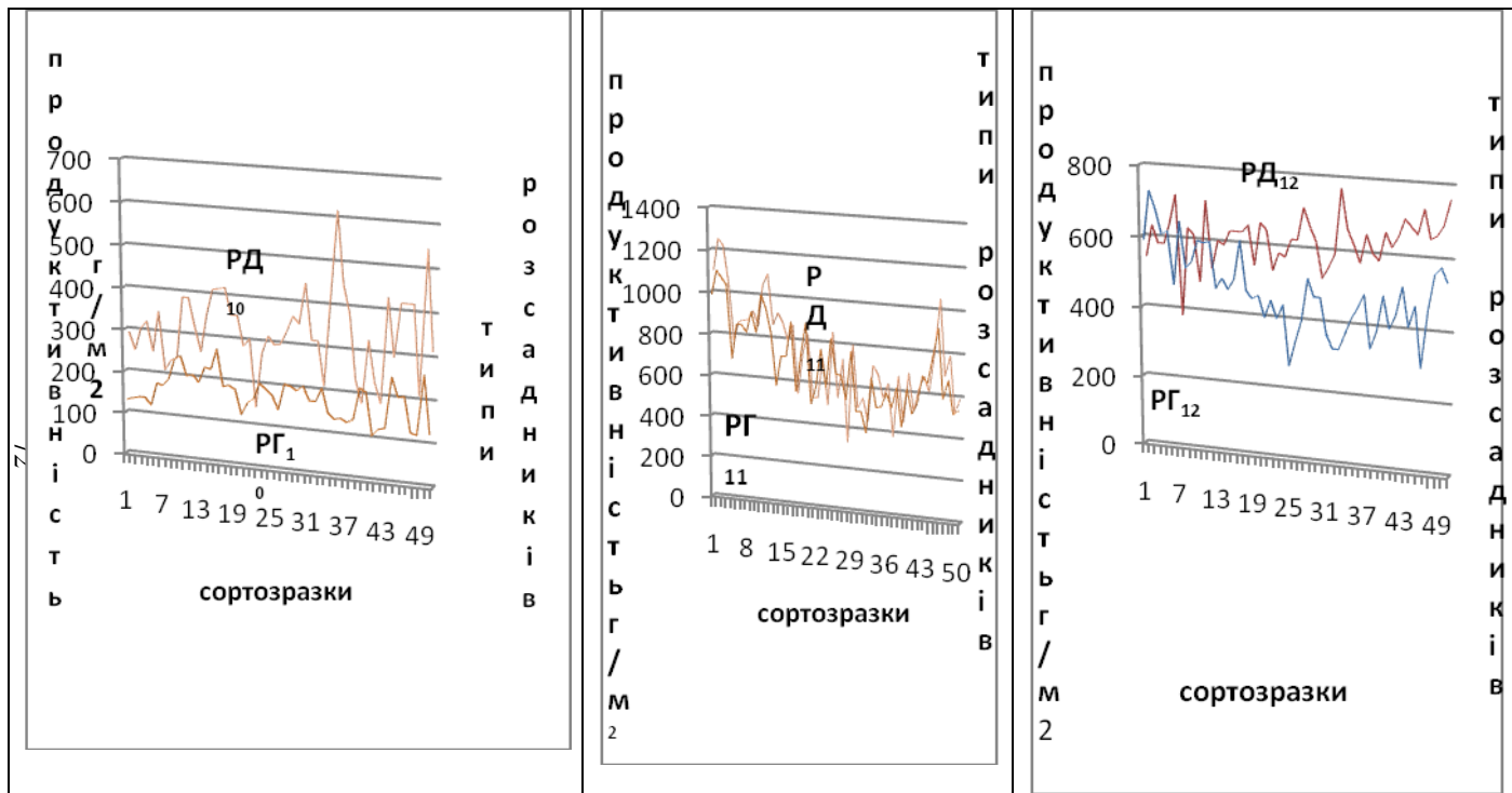
Рис. 6. Параметрична характеристика ступеню селекційного диференціалу зразків жита озимого за насінневою продуктивністю в розсадниках гібридизації (РГ) та елітних доборів (РД), 2010-2012 рр.
