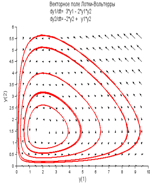
Рис.7. Осцилятор рівнянь Лоткі, Вольтерри у вигляді геометричних областей для нелінійного аналізу взаємозв'язку ознак (у нашому випадку КНБ-МНБ) у зразків пелюшки (на базі програми Scilab), 2009-2012 рр.
