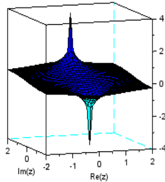
Рис.4. Геометрична модель глобальної стійкості квадратичних моделей загального вигляду на конусі, яка відображає достатні умови існування нетривіального конуса асимптотичної стійкості систем з одним із рівнянь вольтеррівського вигляду (за Чернишенко В. С)
