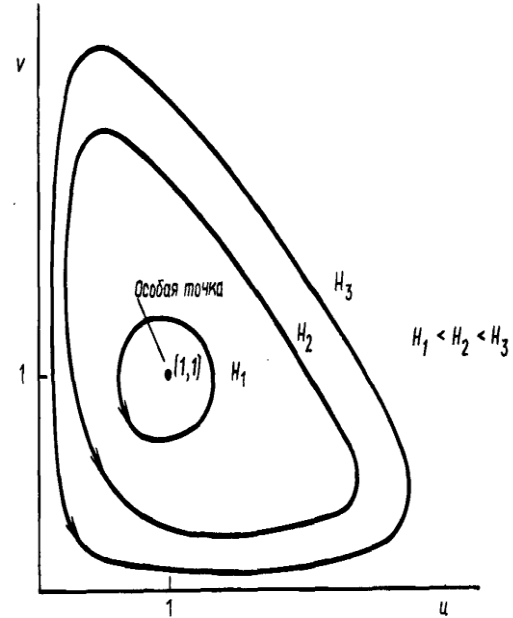
Рис.8. Теоретичні області замкнених траєкторій біологічного осцилятора нелінійної взаємодії факторів, у т.ч. особливі крапки (за Маррі Дж., 1983). au + v - \ln(u^a v) = H = \text{const}
