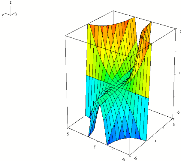
Рис. 1. Теоретична поверхня дизруптивного (розривного) добору за алгоритмом П. Ф. Рокицького та В. К. Савченко, 1975 р. Z ( ^{\wedge}q ) - максимізований параметр ознаки в системі взаємодії частот генів при доборі за формулою z=xy^2*0.5/1-0,5*(1-y^2) , XY ( pq ) - частота алельних станів генів по контролю ознаки, в т. ч. маси 1000 насінин
