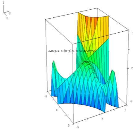
Рис.3. Поверхня моделі (з використанням реальних індексів та частот генів) поліпшуючого добору в гетерозиготних популяціях зразків жита озимого (при доборі на користь гетерозигот) за алгоритмами П. Ф. Рокицького, 1975 р., для пошуку оптимізованих співвідношень параметрів компонентних ознак при формуванні максимуму комплексної ознаки шляхом активного використання даної моделі в режимі он-лайн.
