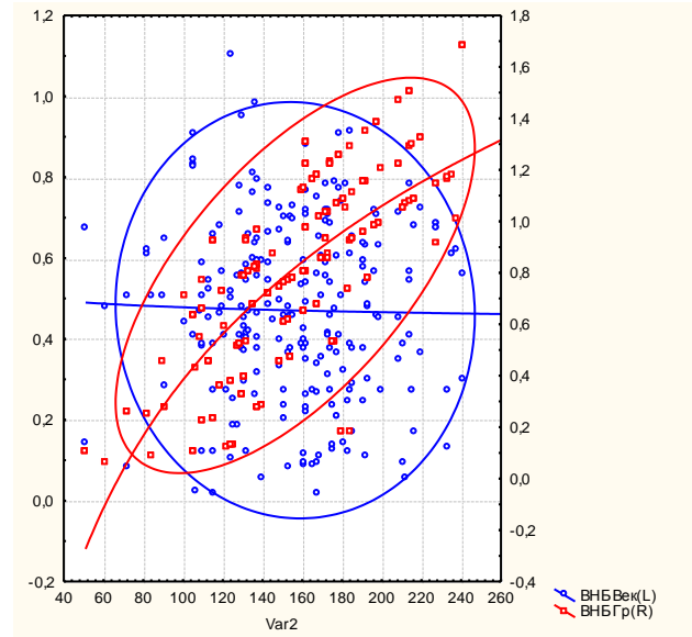
Рис. 10. Диференціація зразків пелюшки зернофуражного (Древлянська, овал) та укісного (Вектор, круг) напрямів використання за комплексною ознакою ВНБ (маса насіння в одному бобі) на фоні компонентної ознаки МТН (маса 1000 насіння), генеалогічна історія сімей, 2003-2011 рр.
