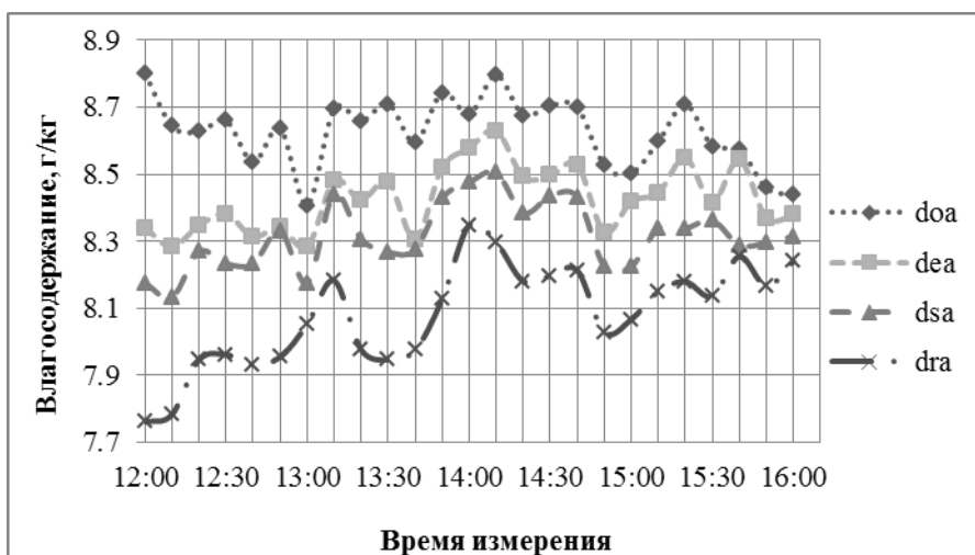
Рисунок 4 – Экспериментальные данные по влажосодержанию
