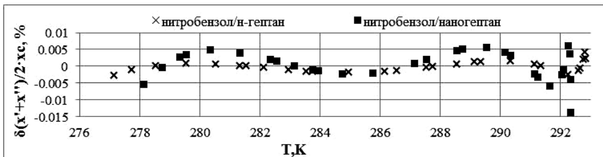
Рисунок 9 – Отклонения экспериментальных данных \delta(x'+x'')/2 \cdot x_c , % от рассчитанных по уравнению (4) концентраций нітробензола для смеси нітробензол/гептан і нітробензол/наногептан
