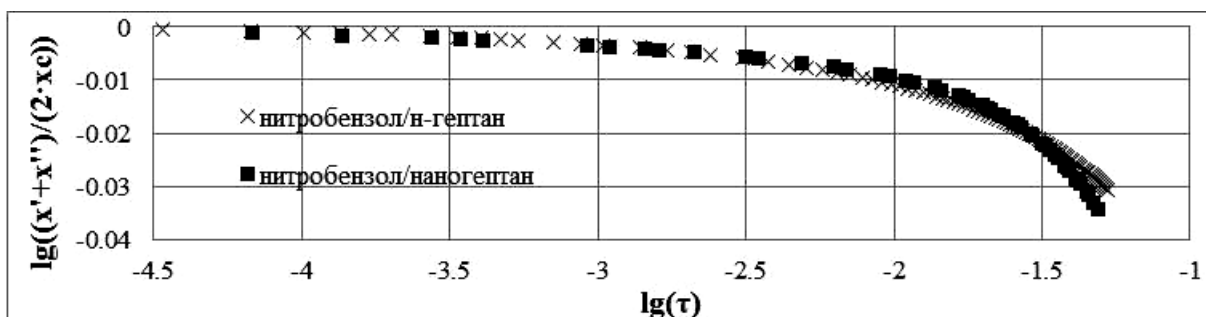
Рисунок 10 – Прямолинейный диаметр в логарифмических координатах для систем нітробензол/н-гептан і нітробензол/наногептан.
