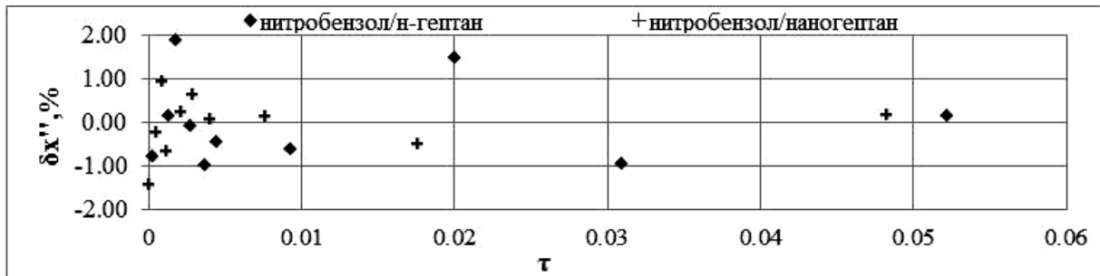
Рисунок 7 – Относительные отклонения экспериментальных значений концентраций нитробензола
