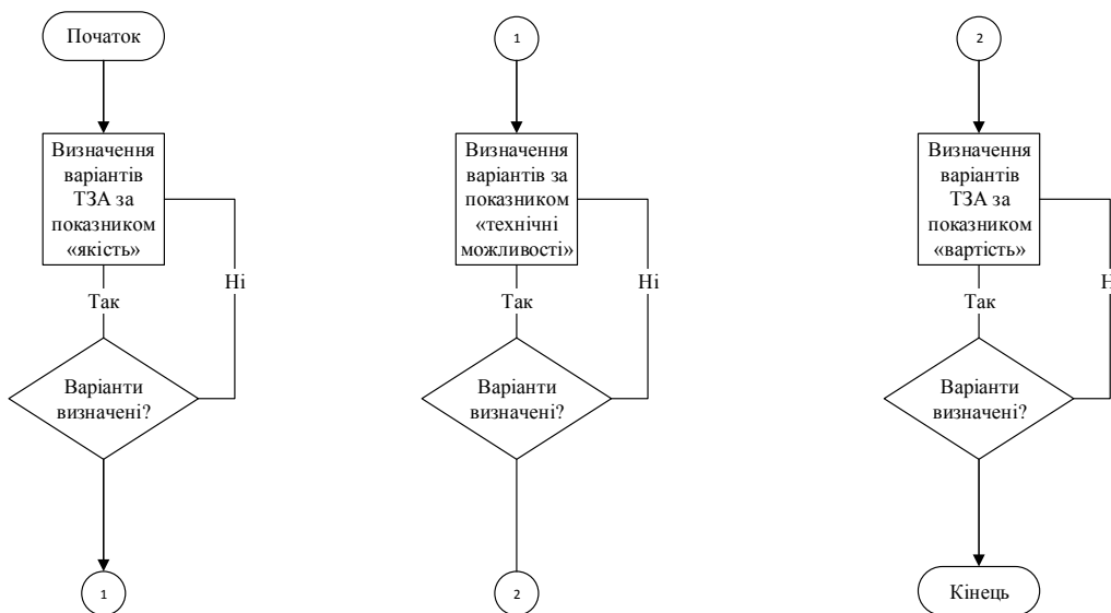
Рис. 1. Загальний вигляд алгоритма вибору технічних засобів автоматизації
