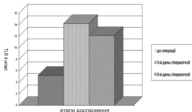
Рис. 1. Динаміка рівня TLR-4 в крові у пацієнтів в залежності від терміну розвитку гіпералгезії
