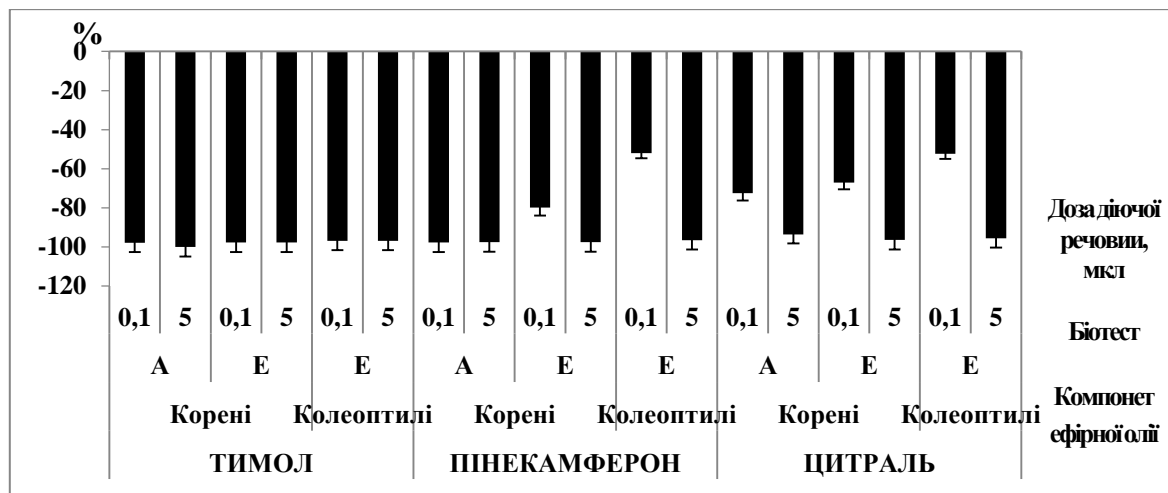
Рис. 5. Вплив деяких складових ефірних олій монарди двійчастої (тимол), змієголовника молдавського (цитраль), гісопа лікарського (пінекамферон) на ріст біотестів. Примітка: 0,1; 5 мкл. – доза діючої речовини на чашку Петрі
