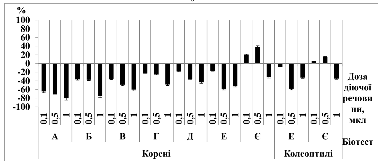
Рис. 4. Вплив ефірної олії на ріст біотестів: а – монарди двійчата; б – змієголовник молдавський; в – гісоп лікарський; А – крес-салат, Б – щиряця хвостата, В – редис посівний, С – ріпак озимий, Д – горох посівний, Є – пшениця озима, Е – ячмінь ярий; 0,1; 0,5; 1,0 мкл. – доза діючої речовини на чашку Петрі
