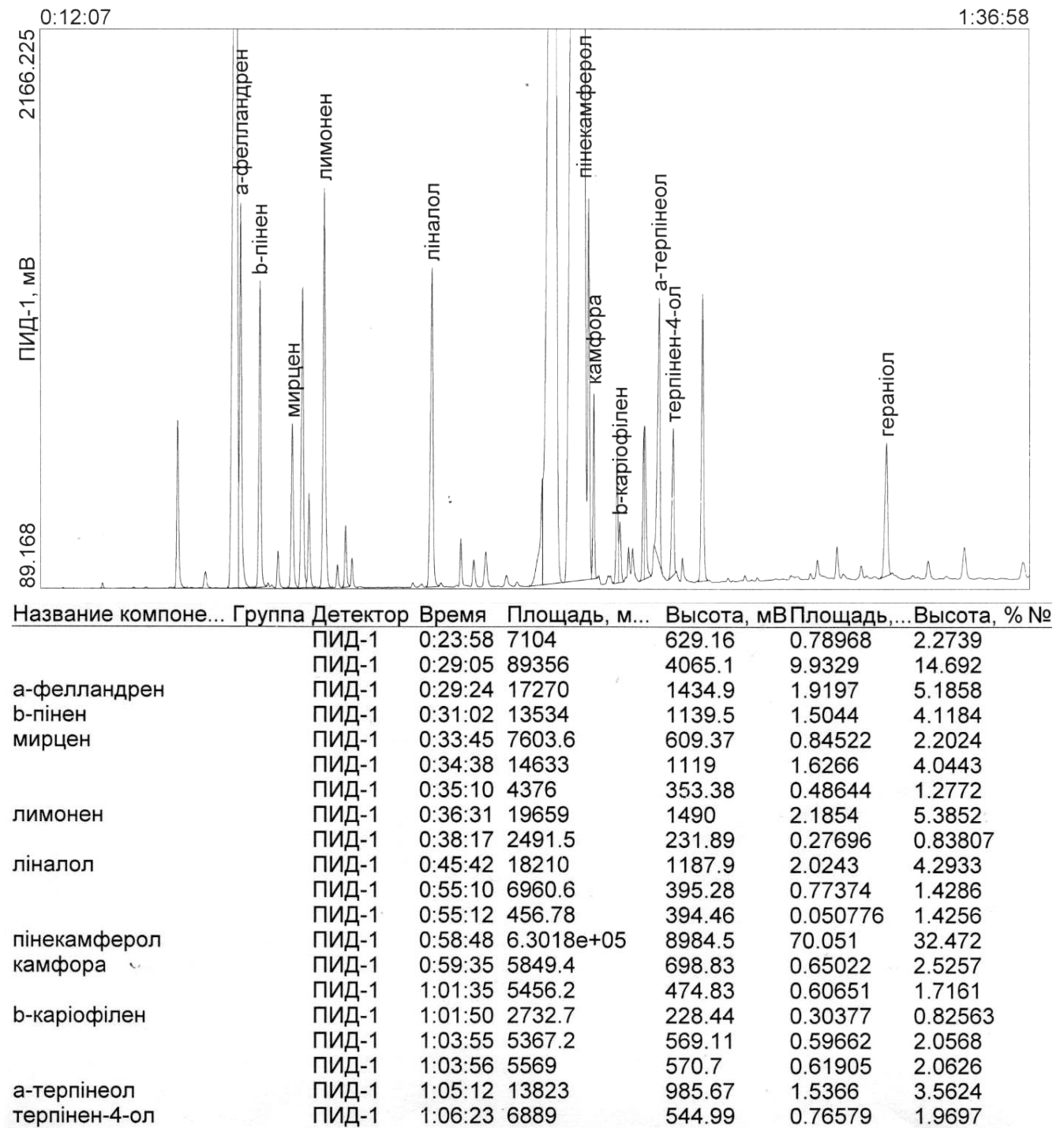
Рис. 1. Хроматограма ефірної олії гісопа лікарського
