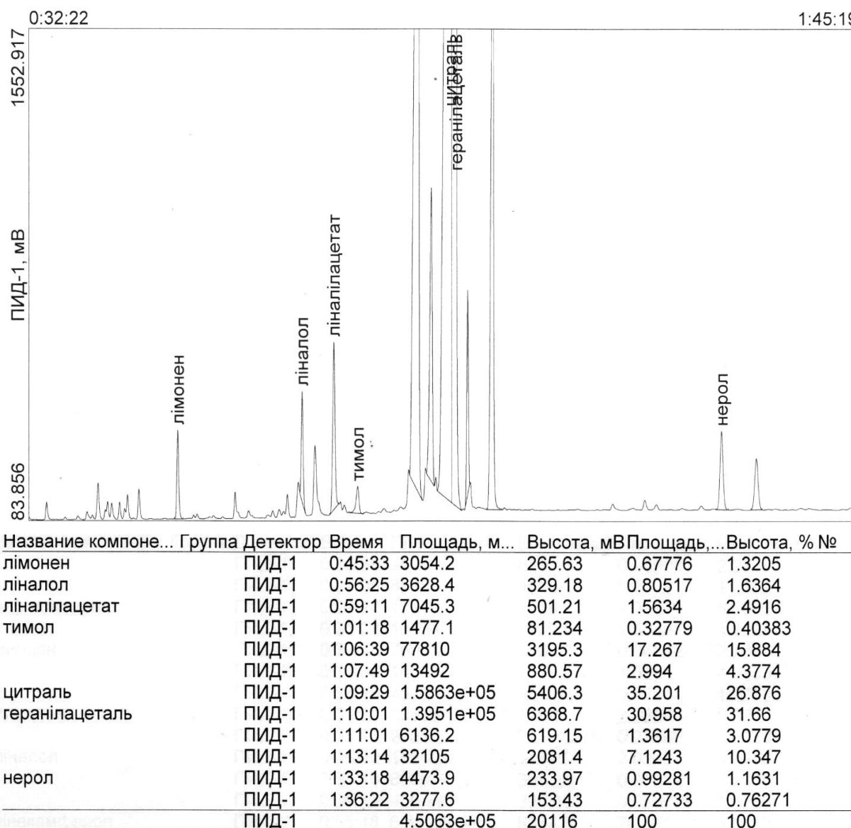
Рис. 2. Хроматограма ефірної олії змієголовника молдавського
