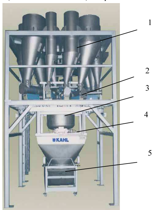
1 – наддозаторні бункери; 2 – живильники; 3 – ваговий дозатор; 4 – оперативний бункер; 5 – конвеєр
