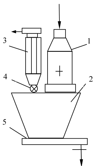
1 – молоткова дробарка; 2 – оперативний бункер; 3 – точковий фільтр; 4 – шлюзовий затвор; 5 – транспортер
