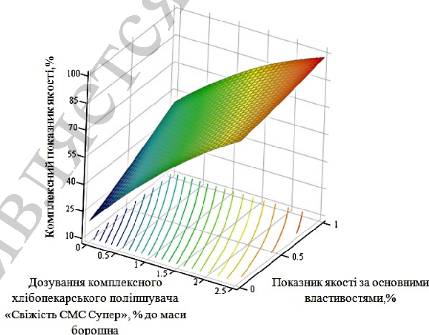
Рис. 2. 3D графік залежності комплексного показника якості від дозування комплексного хлібопекарського поліпшувача «Свіжість СМС Супер» та хлібопекарських властивостей борошна для борошна середнього за силою
