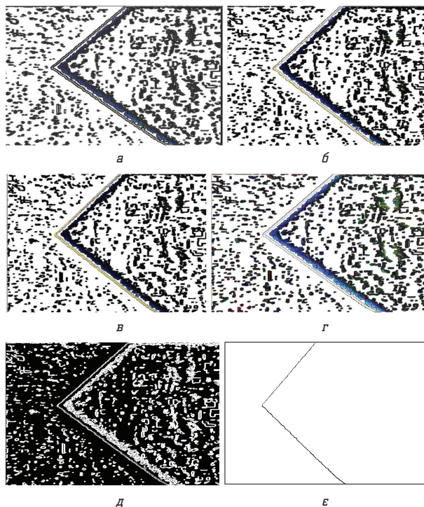
Рис. 7. Зображення з виділеними контурами: а — метод Лапласа, б — метод Собела, в — метод Превітта, г — метод Кірша, д — метод диференційції, е — запропонований метод
