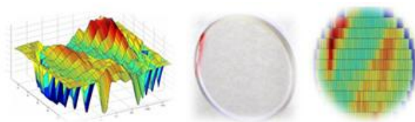
Рис. 3. Приклад нерівномірного розподілу внутрішніх напружень у зразку №3 (модельовання у програмному пакеті MatLab)
