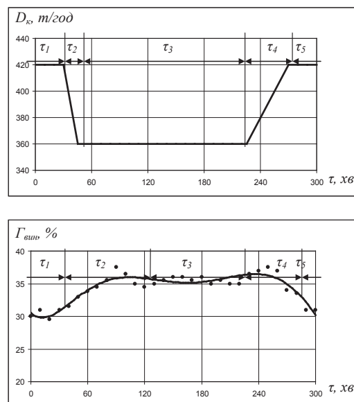
Рис. 1. Залежність механічного недопалу від зміни навантаження
