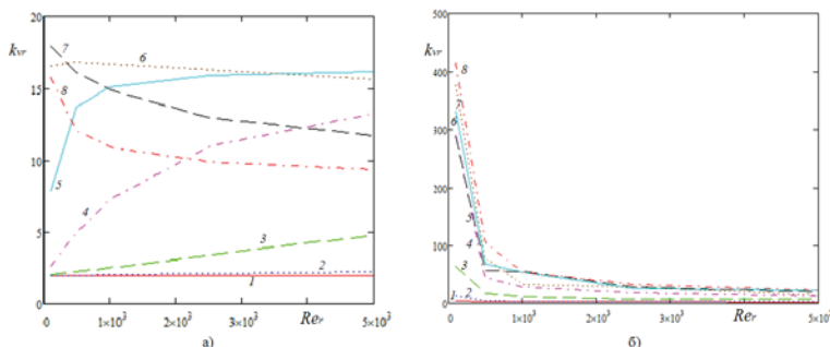
Рис. 2. Значение коэффициента неравномерности k_{vr} для Re_\phi = 10^4 (а) и Re_\phi = 2 \cdot 10^5 : 1 — c = 10^{11} \text{ м}^{-2} ; 2 — c = 10^{10} \text{ м}^{-2} ; 3 — c = 10^9 \text{ м}^{-2} ; 4 — c = 10^8 \text{ м}^{-2} ; 5 — c = 10^7 \text{ м}^{-2} ; 6 — c = 10^6 \text{ м}^{-2} ; 7 — c = 10^5 \text{ м}^{-2} ; 8 — c = 10^4 \text{ м}^{-2}
