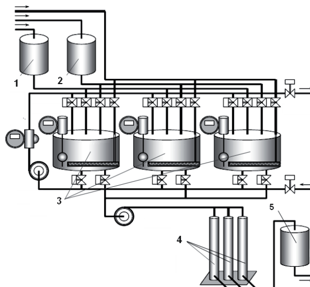
Рис. 1. Періодичний спосіб змішування води і спирту [1]: 1 — ємність для спирту; 2 — ємність для води; 3 — купажні ємності; 4 — вугільні колони; 5 — ємність з готовим продуктом
