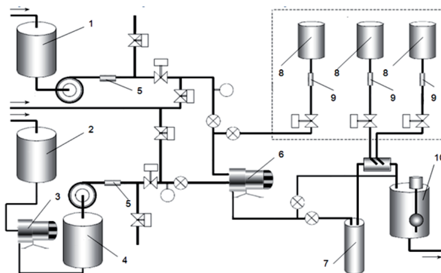
Рис. 2. Схема промислової технологічної лінії для змішування води та спирту в умовах знакозмінних імпульсів тиску: 1 — ємність підготовленої води; 2 — ємність для спирту; 3, 6 — роторно-імпульсійний апарат; 4 — ємність обробленої води; 5 — витратомір; 7 — вугільна колона; 8 — ємності зі смаковими та ароматичними добавками; 9 — витратомір; 10 — ємність готової продукції
