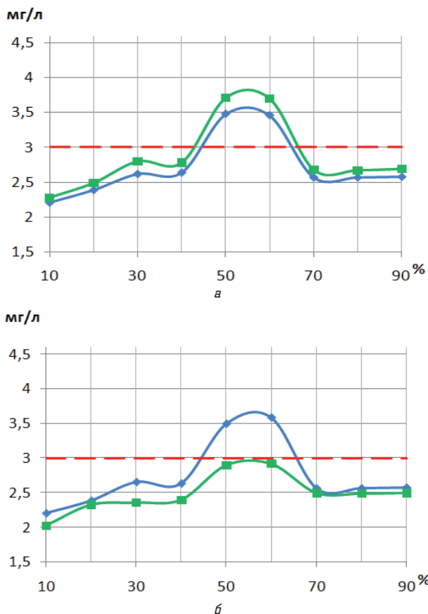
Рис. 3. Вміст ацетальдегіду в сумішах різної концентрації залежно від часу: a — перша година після одержання; б — 24 години після одержання
