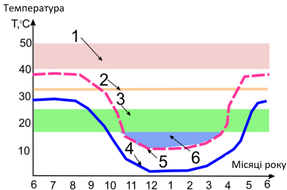
Рис. 3 – Температурні зміни протягом року на території України: 1 – межі допустимих температур у підкостюмному просторі рятувальника (від 40 до 50°C, що відповідає температурі на поверхні тіла рятувальника та внутрішній поверхні одягу); 2 – середньостатистична температура поверхні тіла людини; 3 – межа температур, що є комфортними для людини (від 18 до 25°C); 4 – середньостатистична температура води у водоймищах; 5 – температура в підкостюмному просторі рятувальника; 6 – межа температурних значень, що відповідають умовам охолодження організму рятувальника
