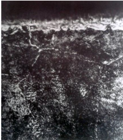
Рис. 1 – Микроструктура покрытия на стали У10 ( \times 600 ) после диффузионного хромирования в смеси №2
