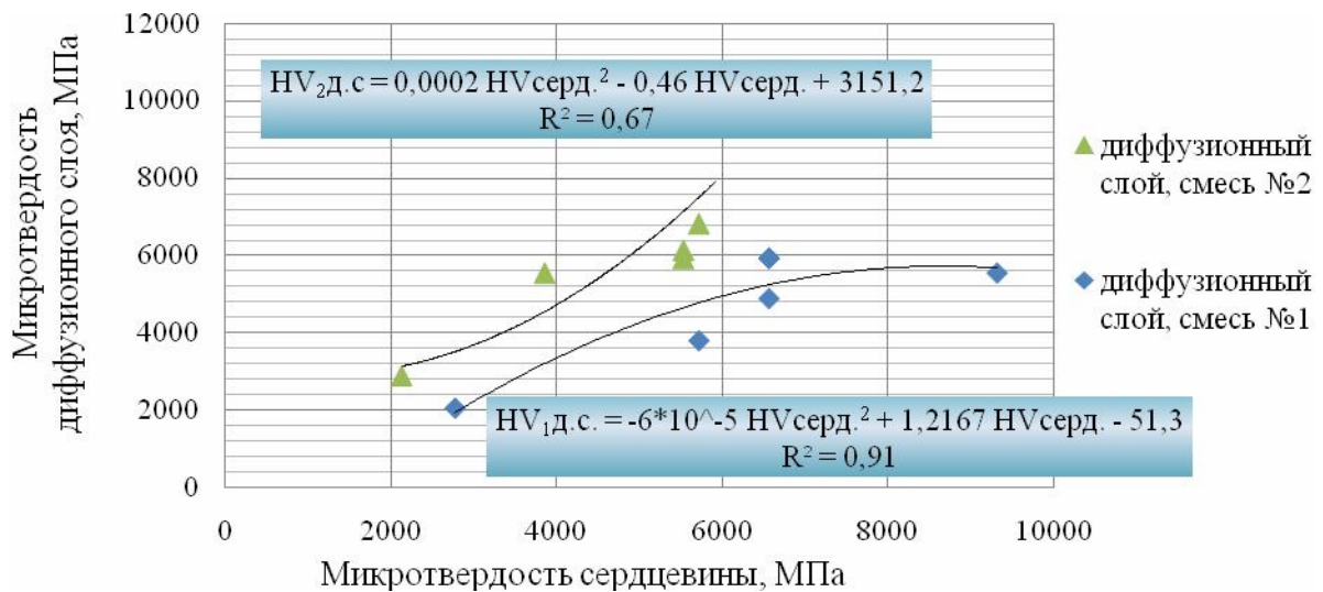
Рис. 8 – Регрессионные модели зависимости микротвердости диффузионного слоя от микротвердости сердцевин
