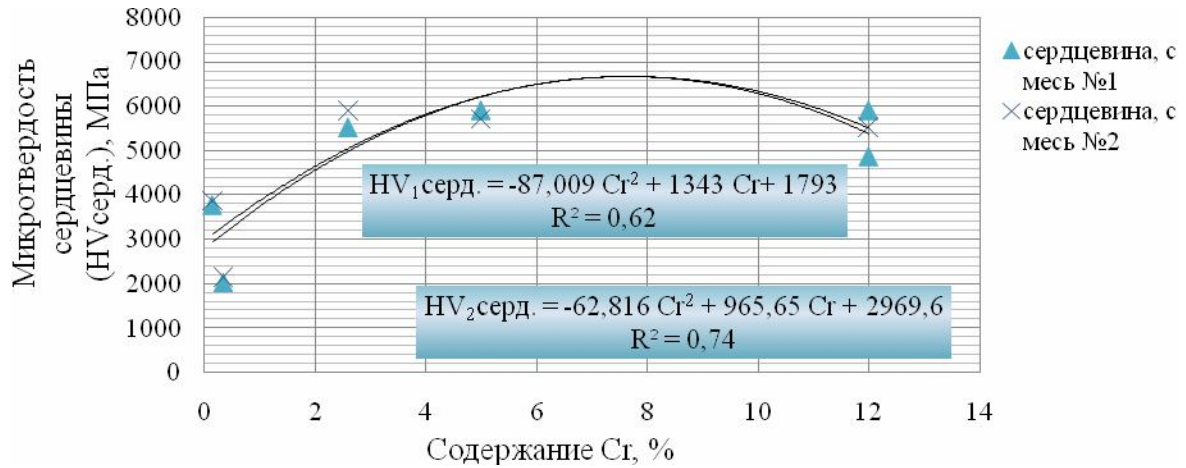
Рис. 7 – Влияние концентрации Cr на микротвердость сердцевин
