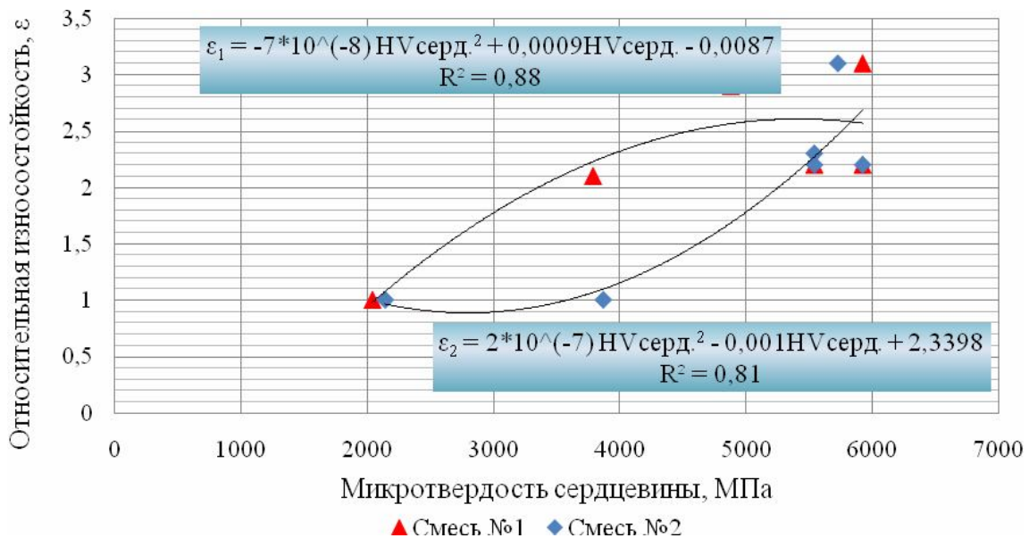
Рис. 10 – Регрессионные модели зависимости относительной износостойкости сталей от микротвердости сердцевины
