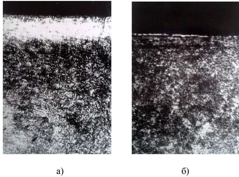
Рис. 3 – Влияние состава насыщающей смеси на толщину слоя карбида хрома стали 3Х2В8, \times 300 : а) смесь №1; б) смесь №2
