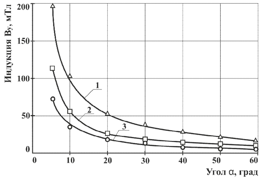
Рис. 6 – Зависимость индукции B_y от угла \alpha при одинаковой плотности тока в электродах ( j=70,8 \text{ A/m}^2 ): 1, 2, 3–диаметры электродов 3, 4, 5 мм
