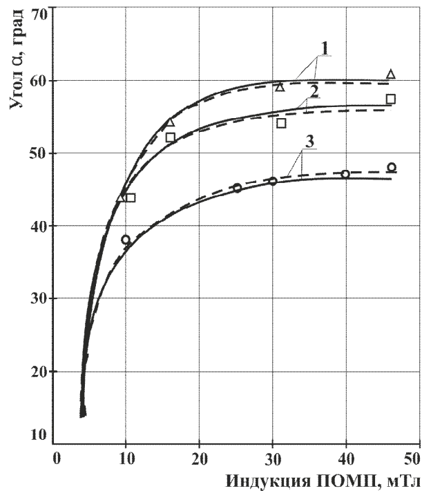
Рис. 2 – Зависимість угла \alpha від індукції ПОМП ( I_n=500 А) для електродів діаметрами: 1 – \Delta – 3 мм, 2 – \square – 4мм, 3 – \circ – 5мм. (прямі лінії – експериментальні дані, пунктирні лінії – розрахункові дані)
