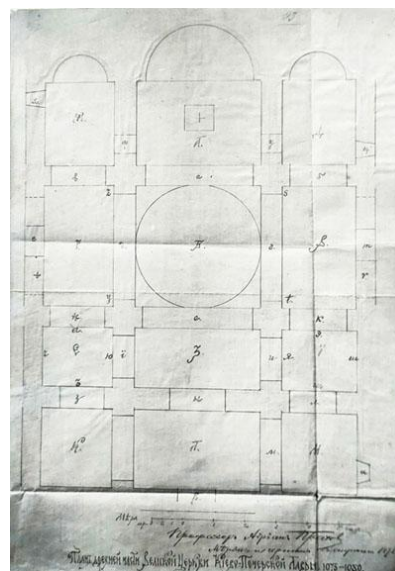
Рис. 1. План давньої частини Великої церкви Києво-Печерської лаври. 1073–1089. Фото креслення, виконаного за розпорядженням А. Прахова в 1893 р. НЗКПЛ
