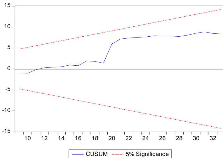
Fig. 1. CUSUM test
