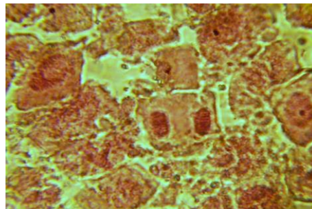
Рисунок 4. Мікроядра у телофазі
